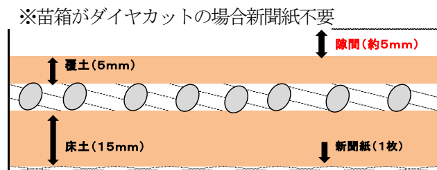
■図1: 播種後の苗箱断面図
